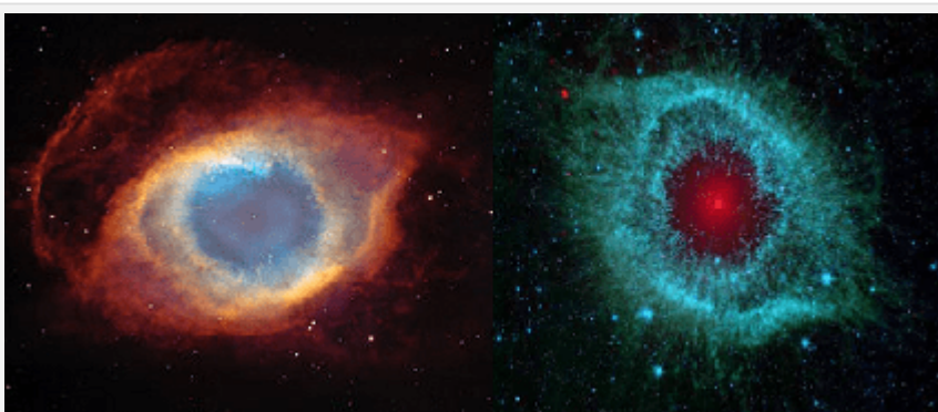
La nebulosa Helix
